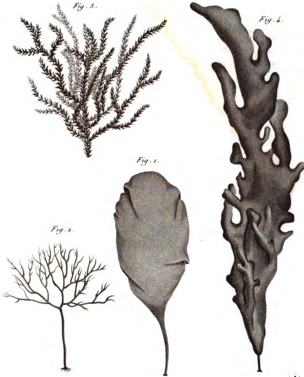
Fig. 1 Ulva caulescens. Fig. 2 Bryopsis balbisiana. Fig. 3 Caulerpa flexilis. Fig. 4 Alujonidium diaphanum.
